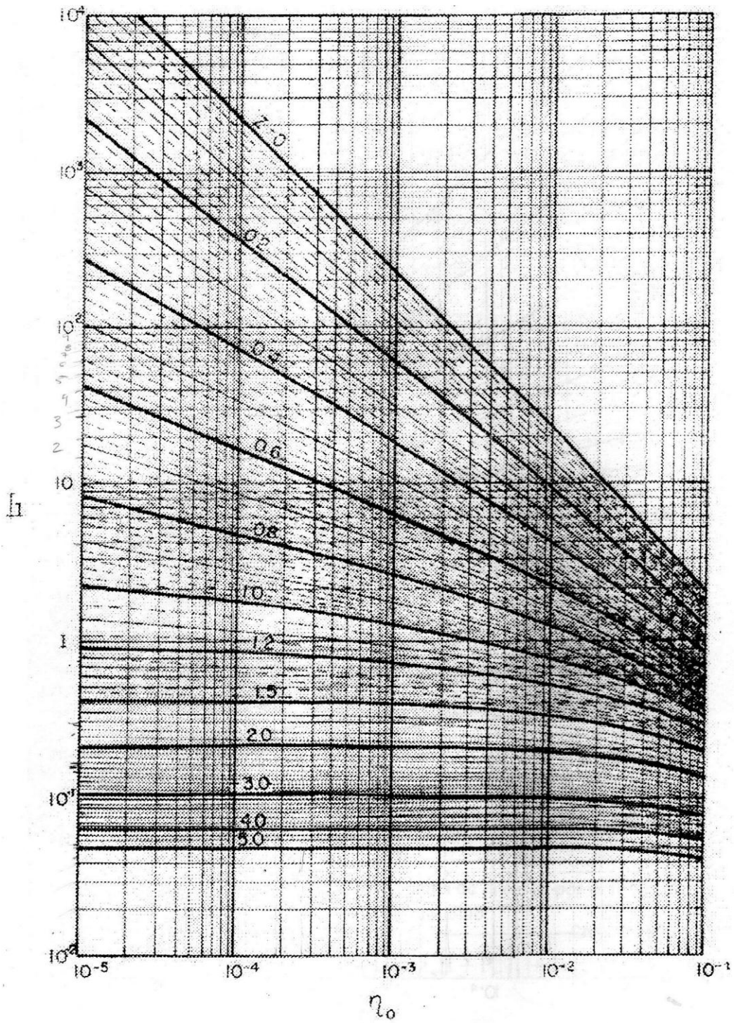
Figura 4.13 Integral I_1 de Einstein, 1950. (Aguirre, 1980).
