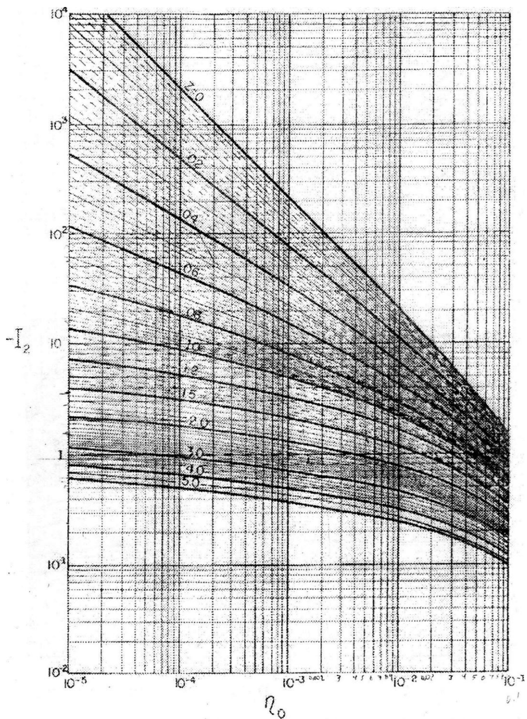
Figura 4.14 Integral I_2 de Einstein, 1950. (Aguirre, 1980).
