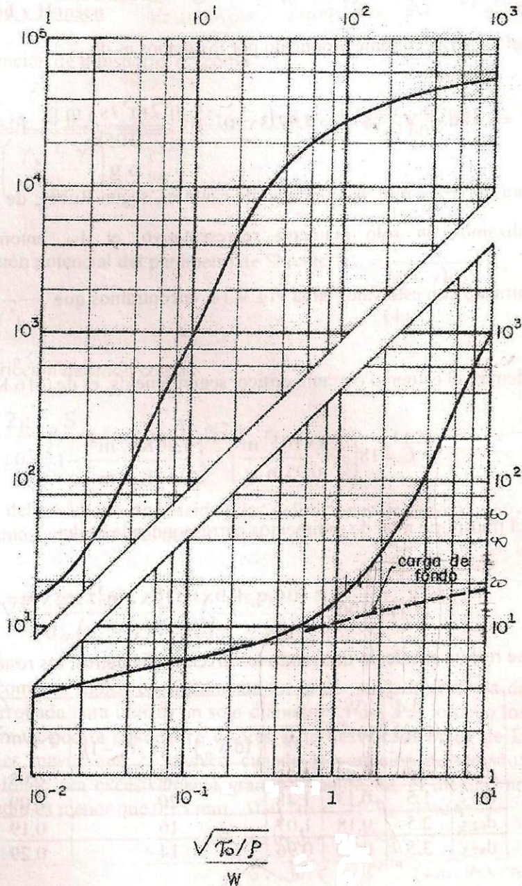
Figura 4.15 Función de arrastre total de sedimentos según Laursen (1958).
