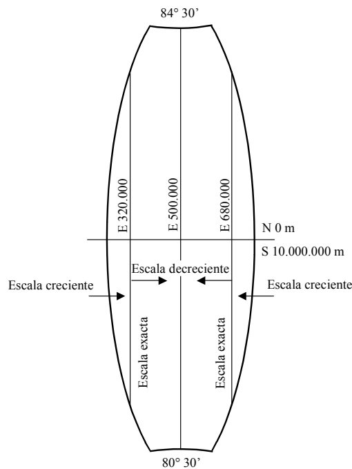
Figura 90. Esquema de zona UTM.
