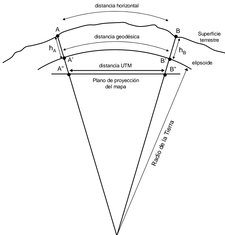
Figura 13. Relación entre distancias horizontales, geodésicas y UTM.
