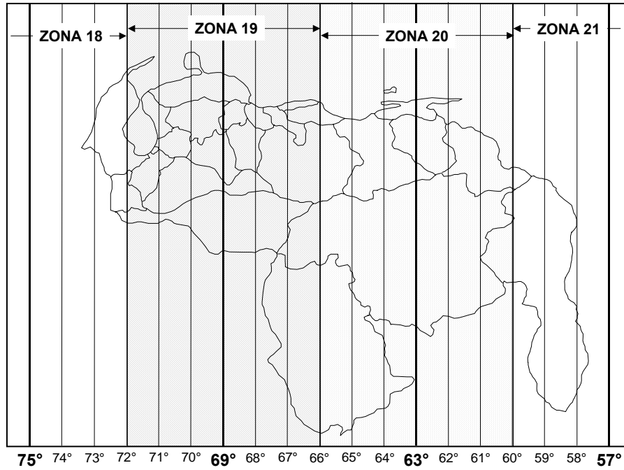
Figura 10. Zonas UTM en Venezuela.
