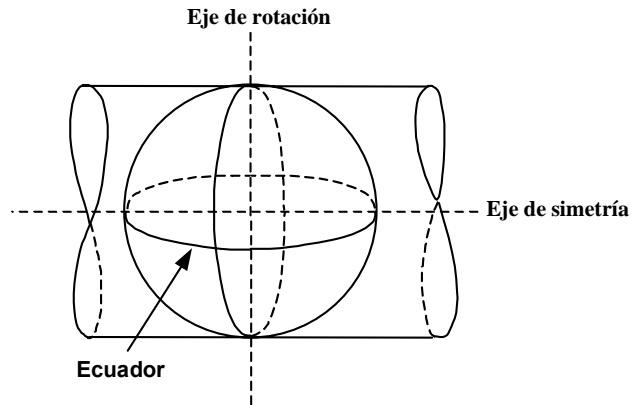
Figura 7. Esquema de la proyección Mercator Transversal.
