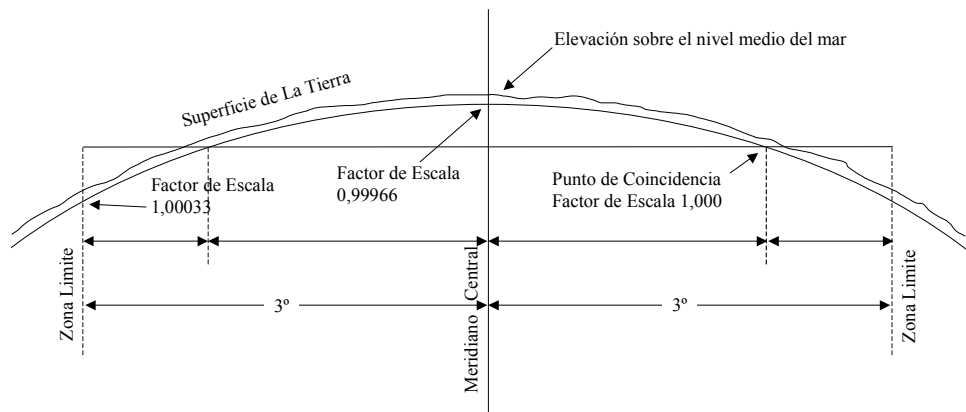
Figura 11. Corte por un paralelo de la proyección UTM
