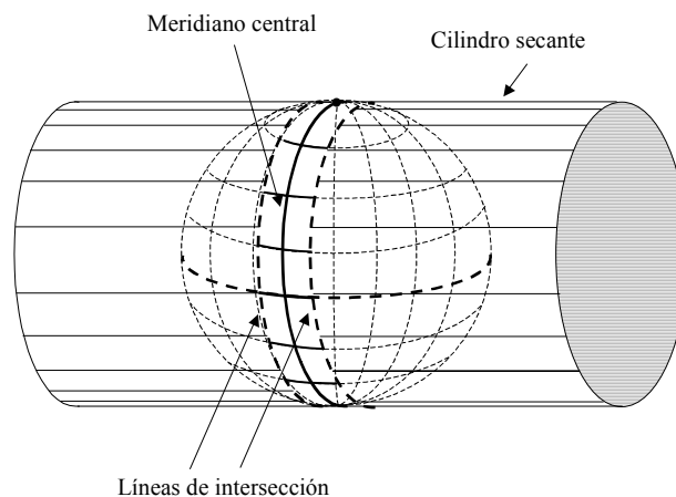
Figura 8. Esquema de la proyección UTM.
