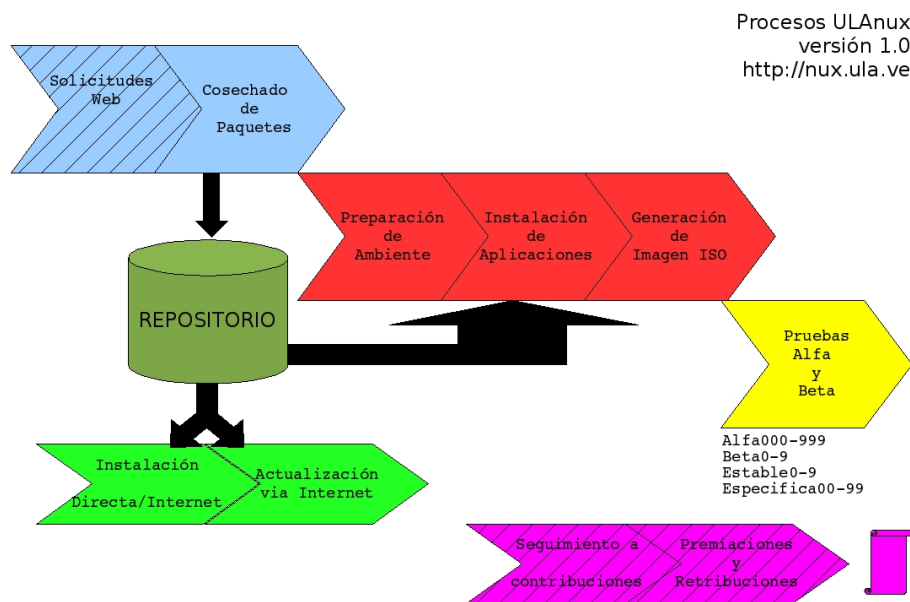
Fig. 1. Los procesos ULAnux
