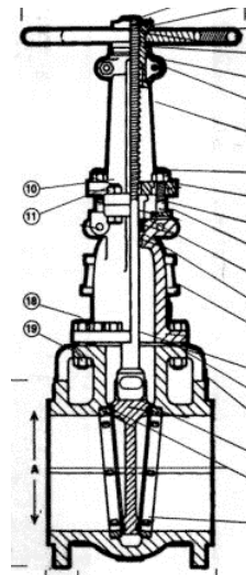
Fig. 4 Válvula de Compuerta
