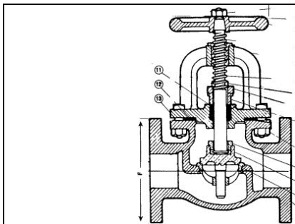
Fig. 2 Válvula de Globo
