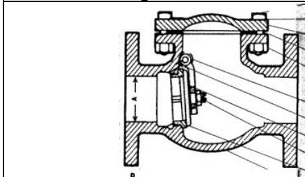
Fig. 3 Válvula de Retención
