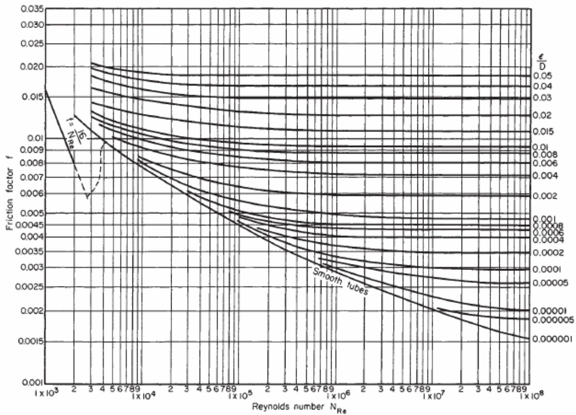
Fig. 1. Diagrama de Moody. Factor de Fricción de Fanning vs. Re [Perry]
