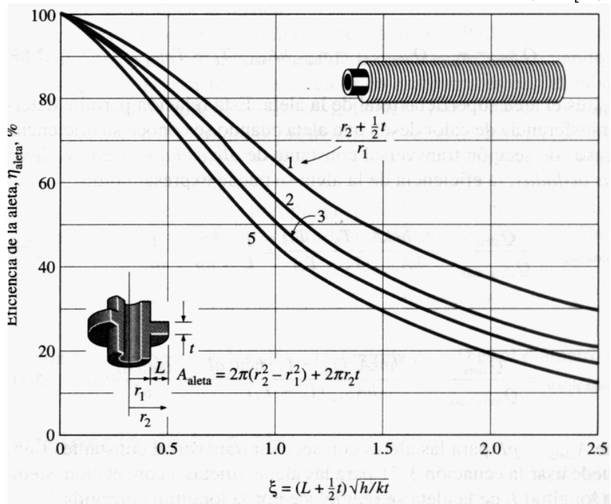
Fig. 2 Eficiencia de aletas circulares de longitud L y espesor constante t
