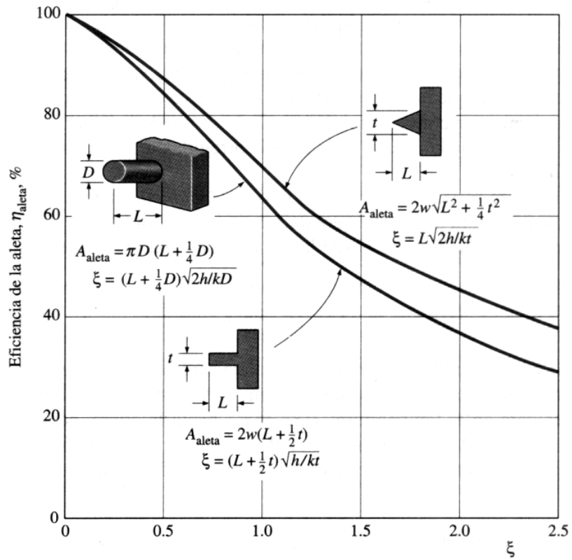
Fig. 1 Eficiencia de aletas rectas (perfiles rectangular, triangular y parabólico).
