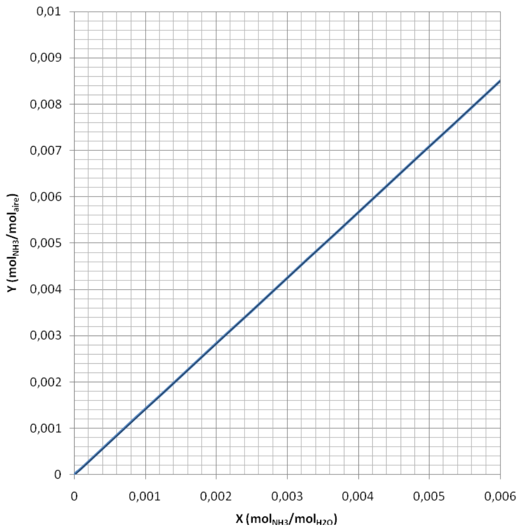
Sistema NH 3 /H 2 O/Aire
