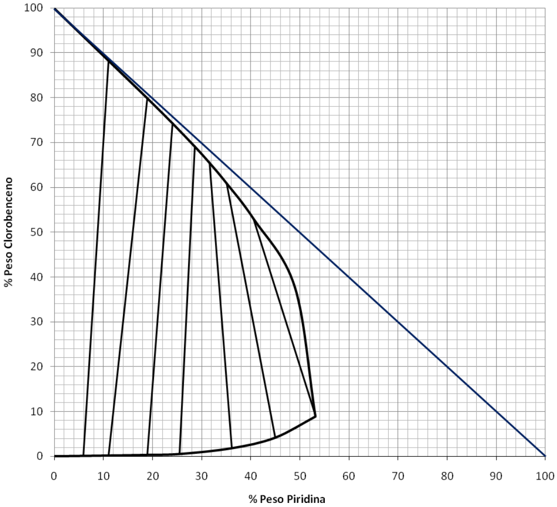
Diagramas del Sistema Piridina-Agua-Clorobenceno (1 atm y 25°C)
