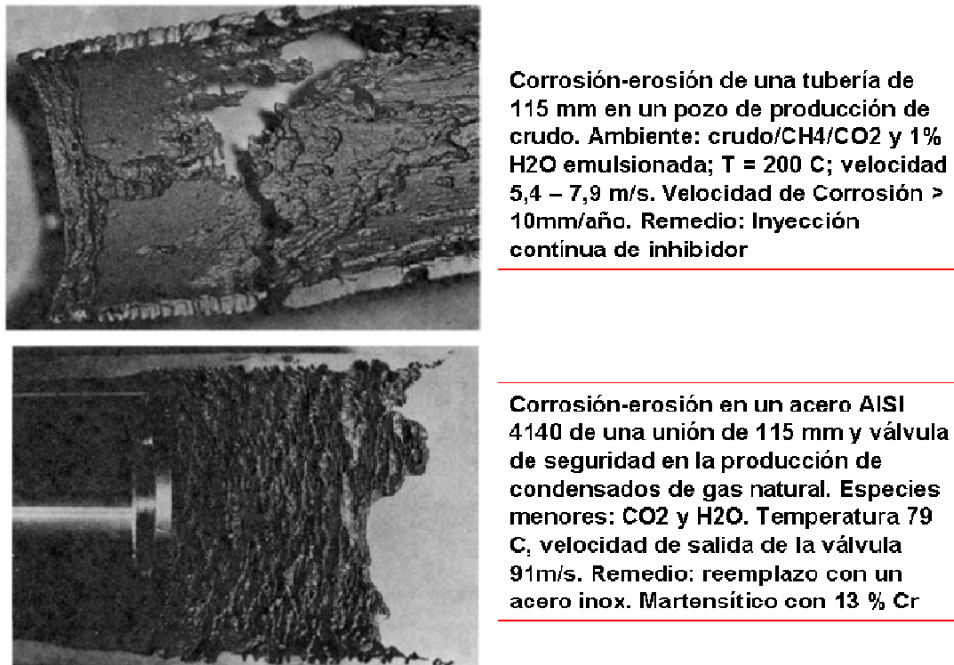
Figura 140 Corrosión- erosión
