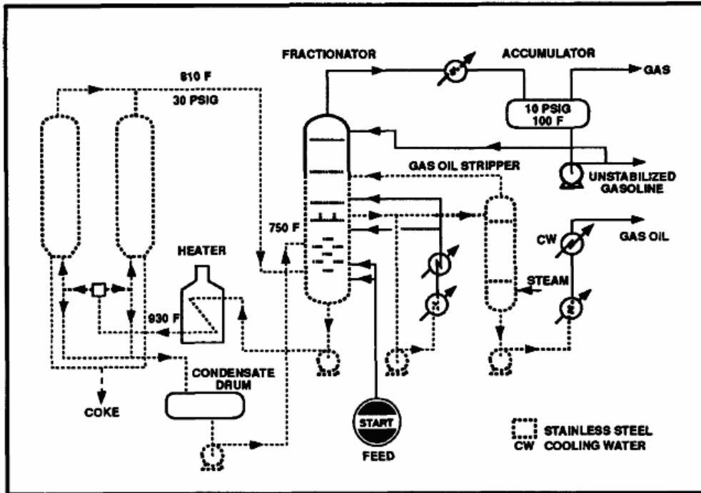
Figura 150 Coquificación retardada
