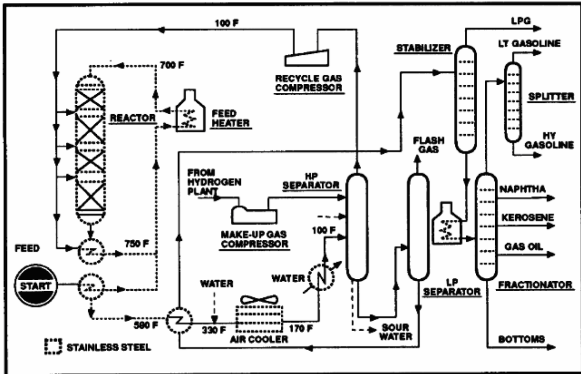
Figura 156 Hidrocrqueo
