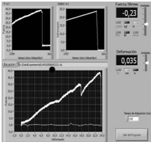
Figura 6. Pantalla de adquisición y procesamiento de datos personalizada según las unidades seleccionadas por el usuario.
