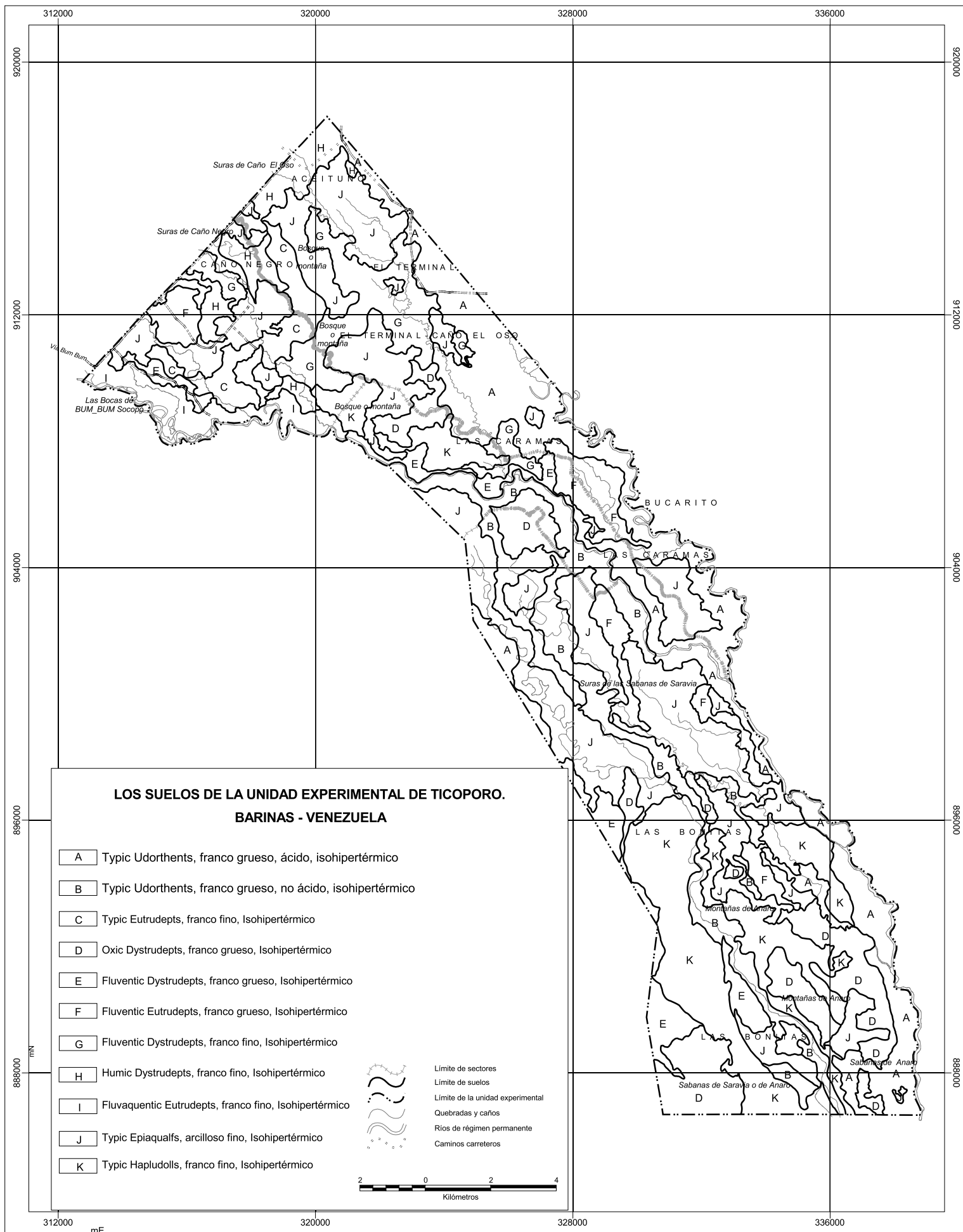
Figura 2. Mapa de los suelos de la Unidad Experimental de Ticoporo. Barinas. Venezuela. Ochoa G., C. Alvarado, J. Oballos, J. Pereira, F. Vargas. 2005.
