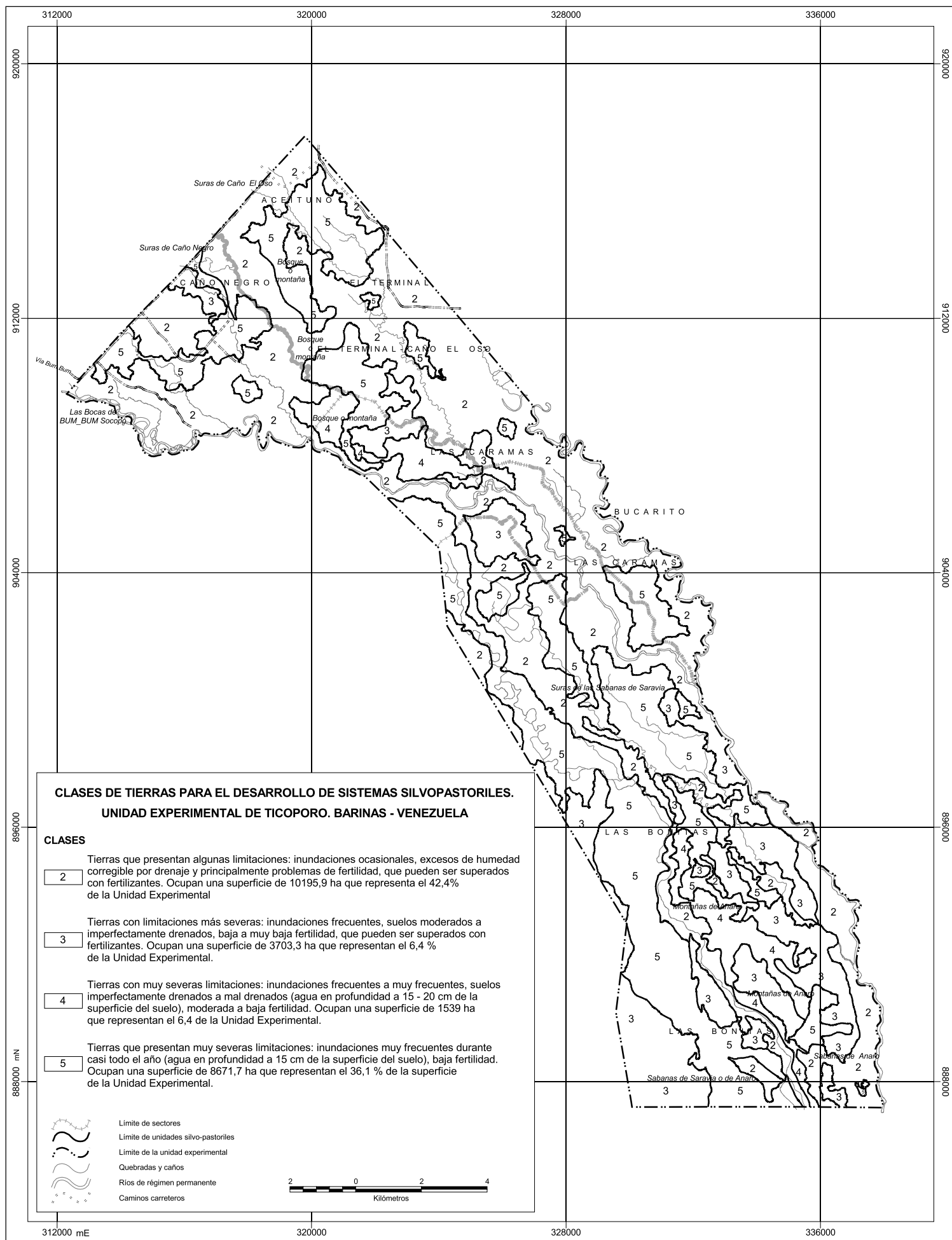
Figura 4. Clases de tierras para el desarrollo de sistemas silvopastorales. Unidad Experimental de Ticoporo. Barinas. Venezuela. Ochoa G., C. Alvarado, J. Oballos, J. Pereira, F. Vargas. 2005.
